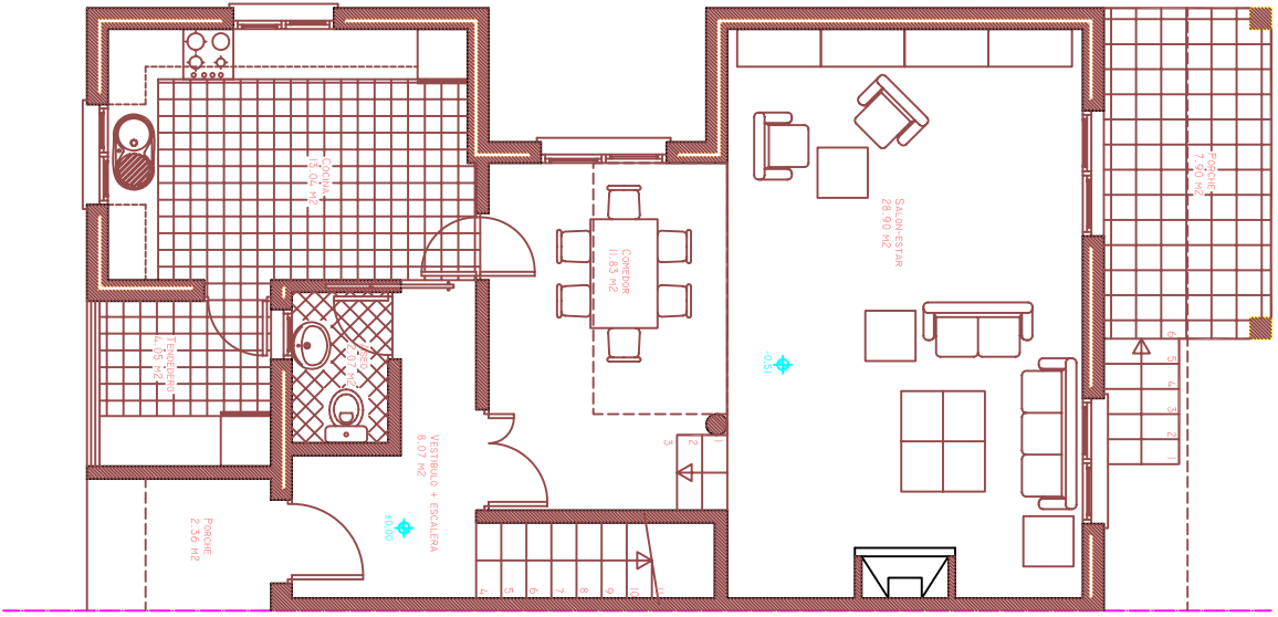
PLANTA BAJA. Sup. construida: 84,98 m 2 VIVIENDAS TIPO 1: PARCELAS Nº 5 Y 10
