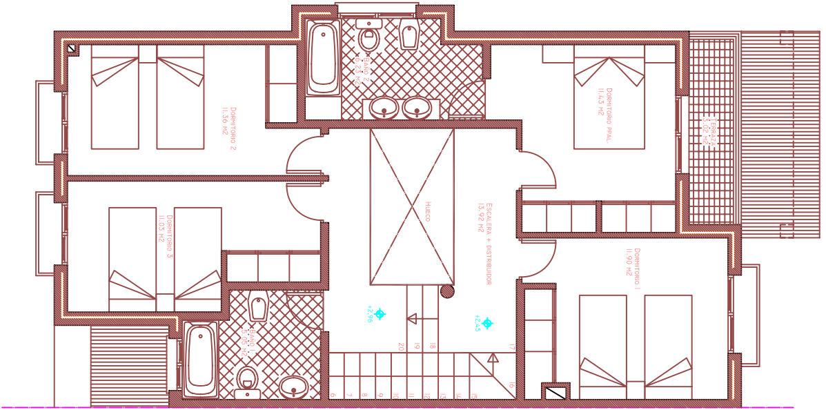
PLANTA ALTA. Sup. construida: 84,26 m 2 VIVIENDAS TIPO 1: PARCELAS Nº 5 Y 10
