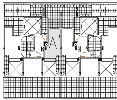
PLANTA BAJOCUBIERTA
