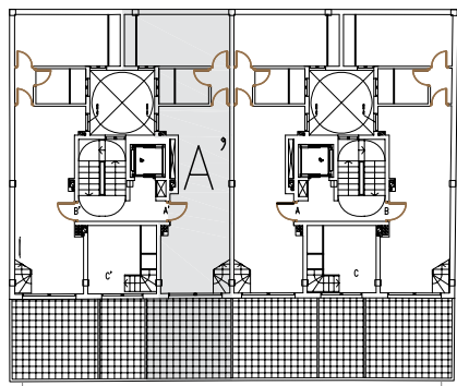
PLANTA ATICO
