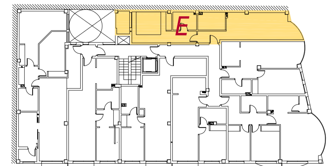
VIVIENDA TIPO E PLANTA SEGUNDA ESCALA: 1/50
