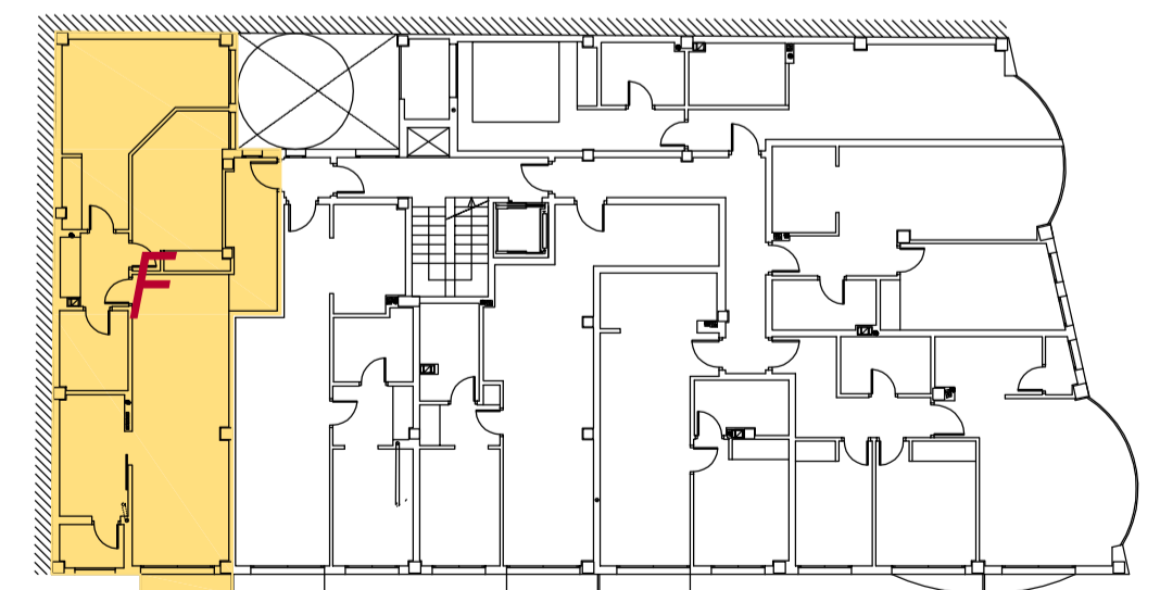
VIVIENDA TIPO F PLANTA SEGUNDA ESCALA: 1/50
